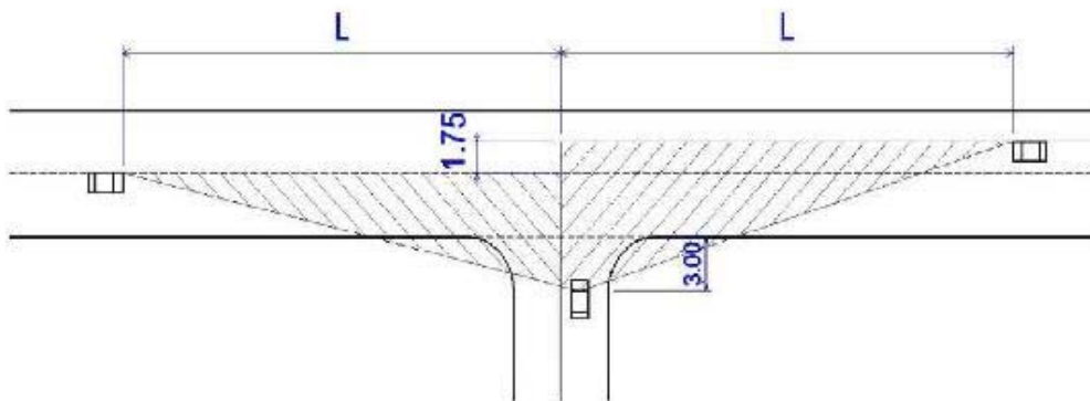
Uzbraukšanas un tuvošanās redzamības brīvlauku pleca garumi (L)
