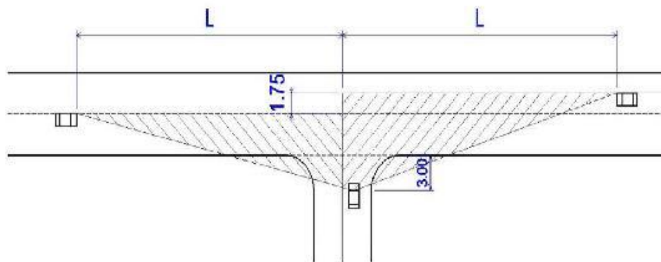
Uzbraukšanas un tuvošanās redzamības brīvlauku pleca garumi (L)
