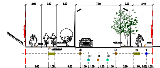
Jaunā iela sarkanās līnijas 20m GRIEZUMS C2-C2
