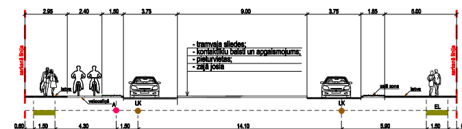
Ojāra Vācieša ielas sarkanās līnijas 30m GRIEZUMS G- G
