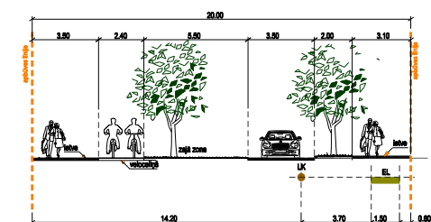
Piebraucamais ceļš 20m GRIEZUMS K-K
