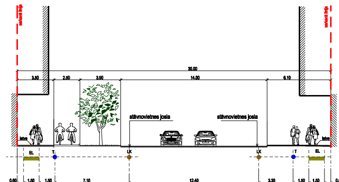
Zemgales iela sarkanās līnijas 30m GRIEZUMS F - F
