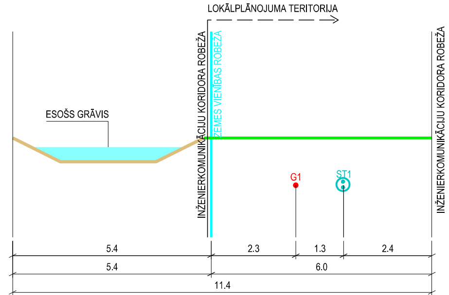
GRIEZUMS 3 - 3 (PLĀNOTĀ INŽENIERKOMUNIKĀCIJU KORIDORA ŠĶĒRSPROFILS)
