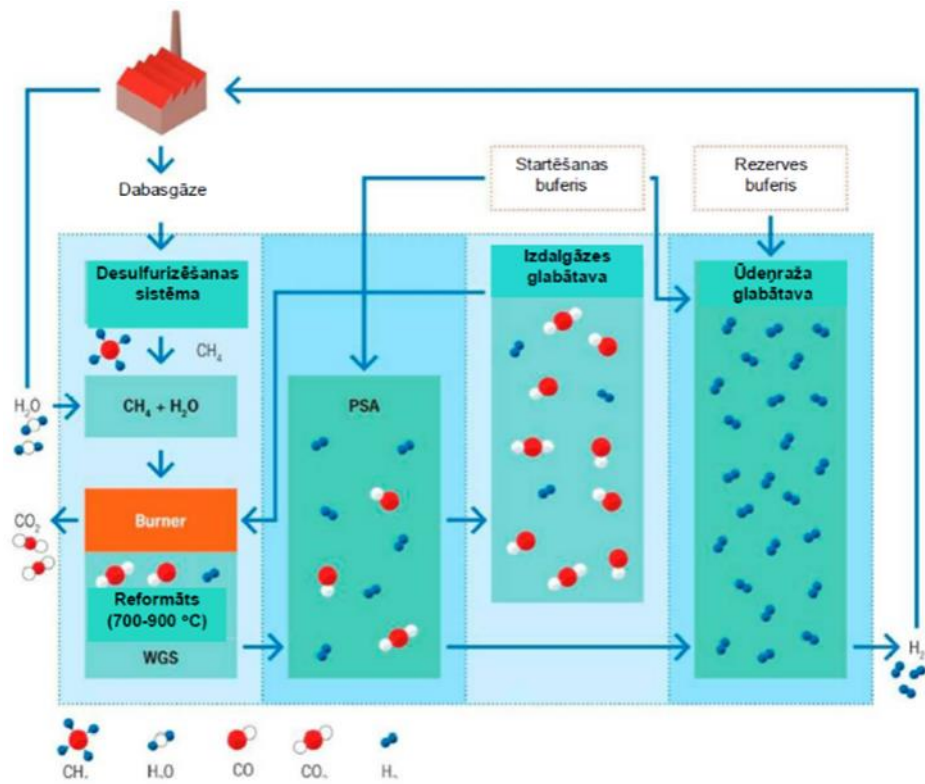
8. Procesa shēma
