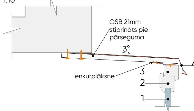
MEZGLS M-119/2
