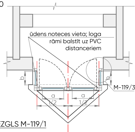
PLĀNA SKATS
