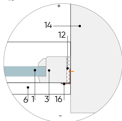
MEZGLS M-103/3
