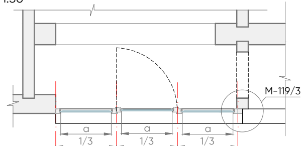
PLĀNA SKATS 1:50
