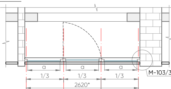
PLĀNA SKATS
