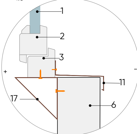
MEZGLS M-103/2
