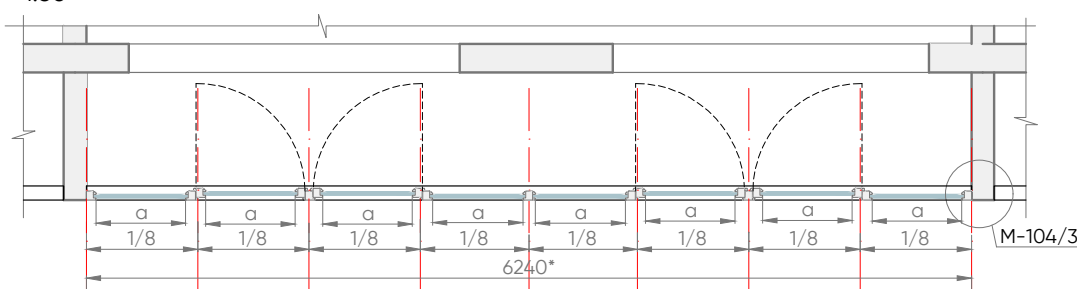
MEZGLS M-104/1
