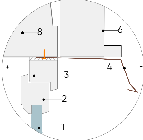
MEZGLS M-119/4 1:5
