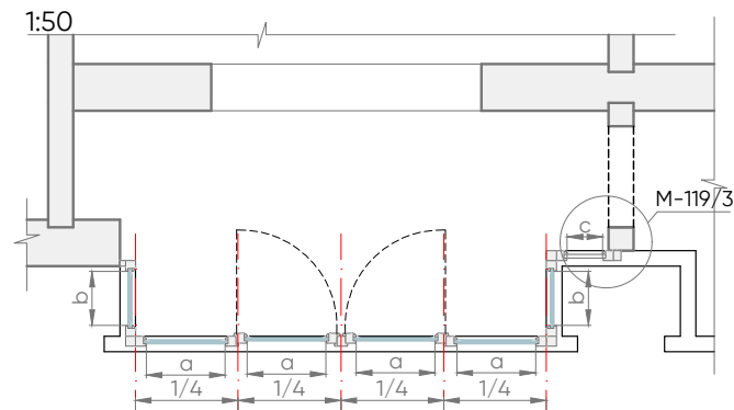
MEZGLS M-119/1
