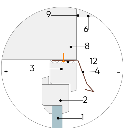
MEZGLS M-103/1
