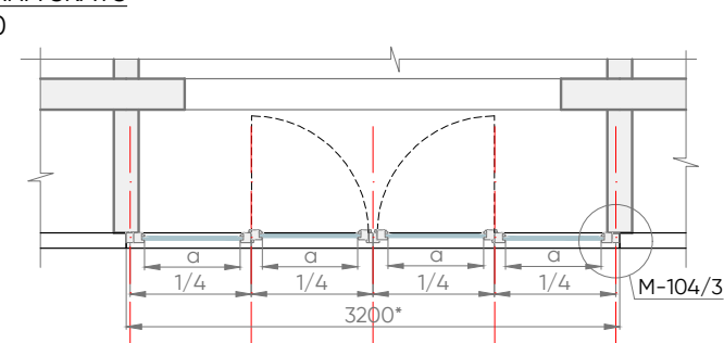
MEZGLS M-104/1
