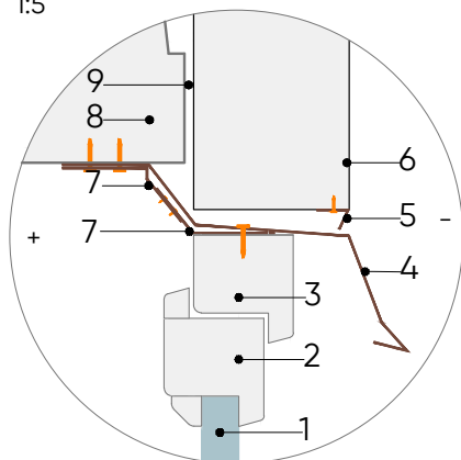
MEZGLS M-467/1
