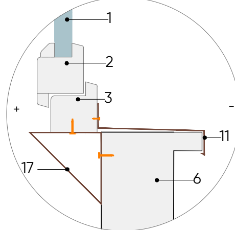
MEZGLS M-119/5 1:5
