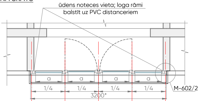
MEZGLS M-602/1
