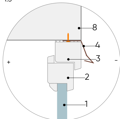
MEZGLS M-104/1
