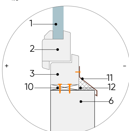
MEZGLS M-104/2
