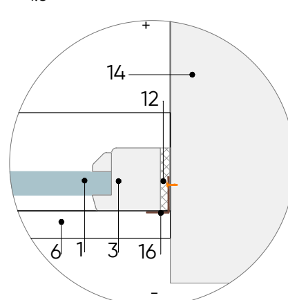
MEZGLS M-103/3
