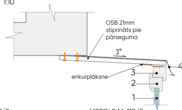
MEZGLS M-119/3
