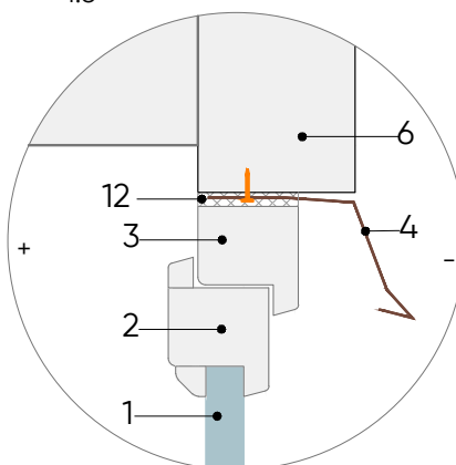
MEZGLS M-103/4
