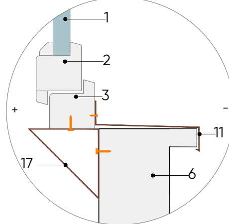
MEZGLS M-119/5
