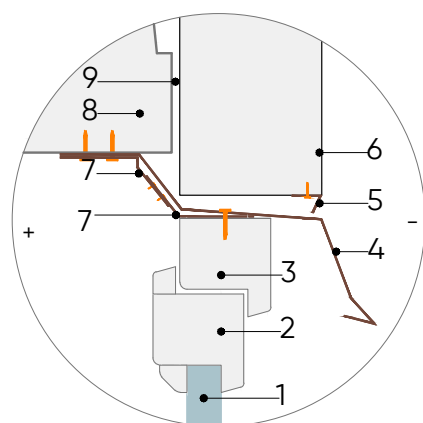
MEZGLS M-119/1
