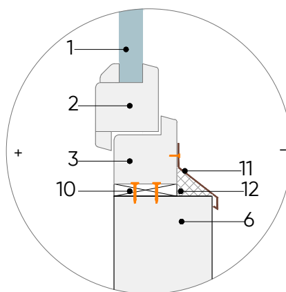
MEZGLS M-119/2
