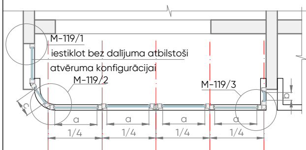
MEZGLS M-119/1
