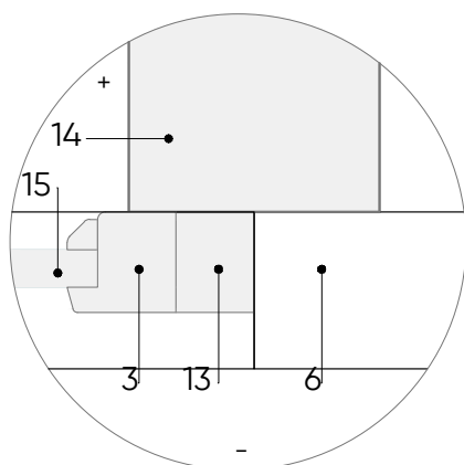
MEZGLS M-119/3 1:5
