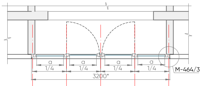
MEZGLS M-464/1
