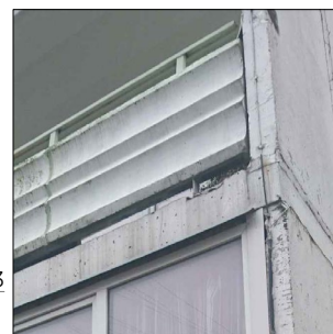
LODŽIJAS MARGAS IZSKATS
