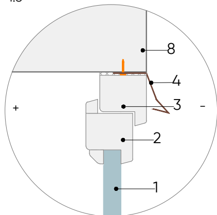
MEZGLS M-464/1
