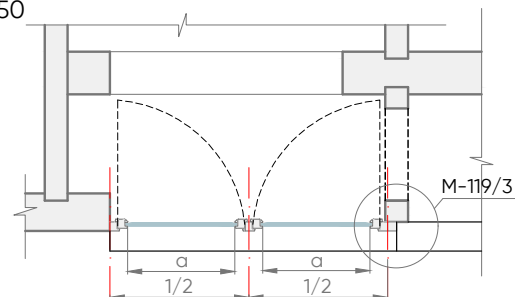
PLĀNA SKATS
