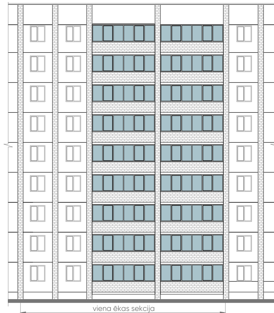
FASĀDES SHĒMA
