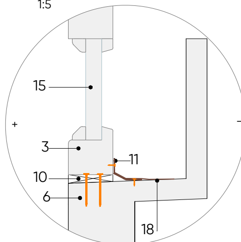
MEZGLS M-119/2
