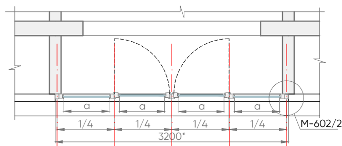
MEZGLS M-602/1
