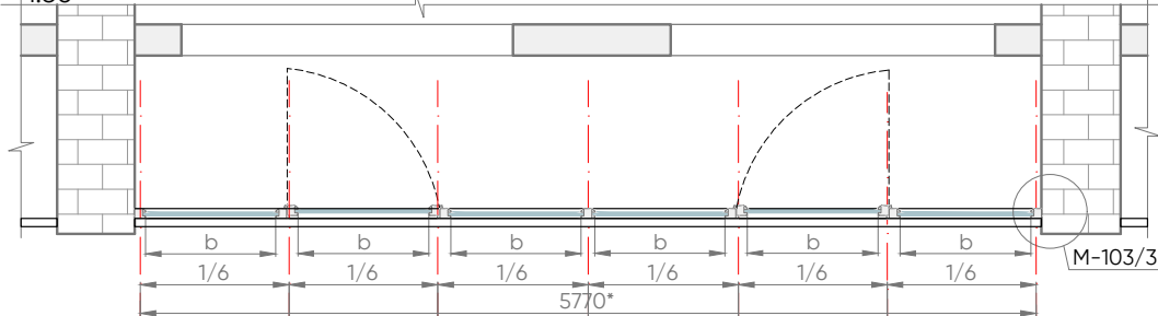
MEZGLS M-103/4
