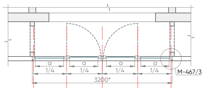
MEZGLS M-467/1
