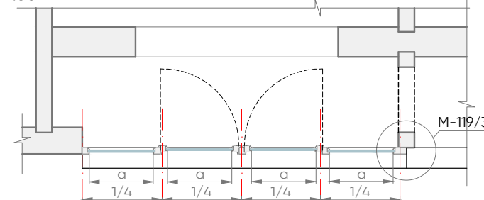
PLĀNA SKATS
