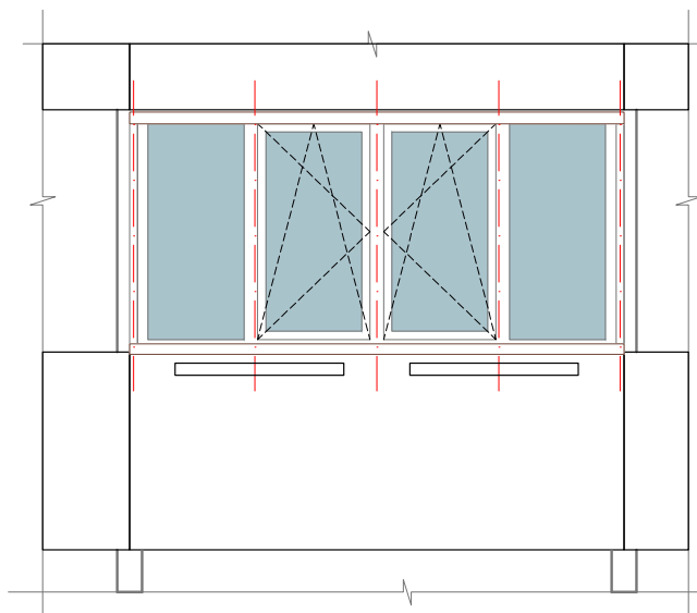
PLĀNA SKATS
