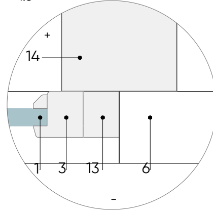
MEZGLS M-104/3 1:5
