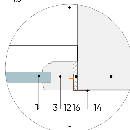
MEZGLS M-104/3
