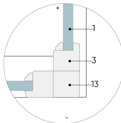
MEZGLS M-119/3
