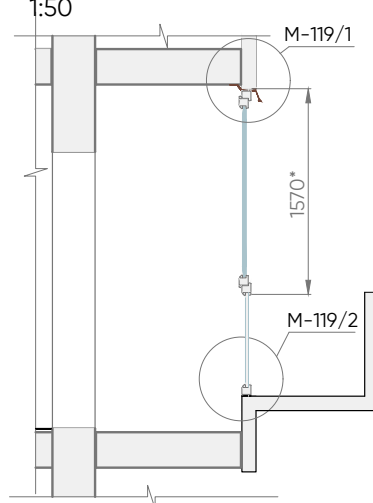
LODŽIJAS MARGAS IZSKATS
