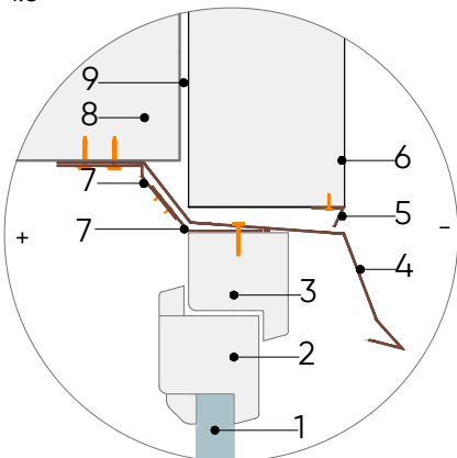
MEZGLS M-104/1 1:5
